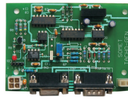
TACHO GEN
